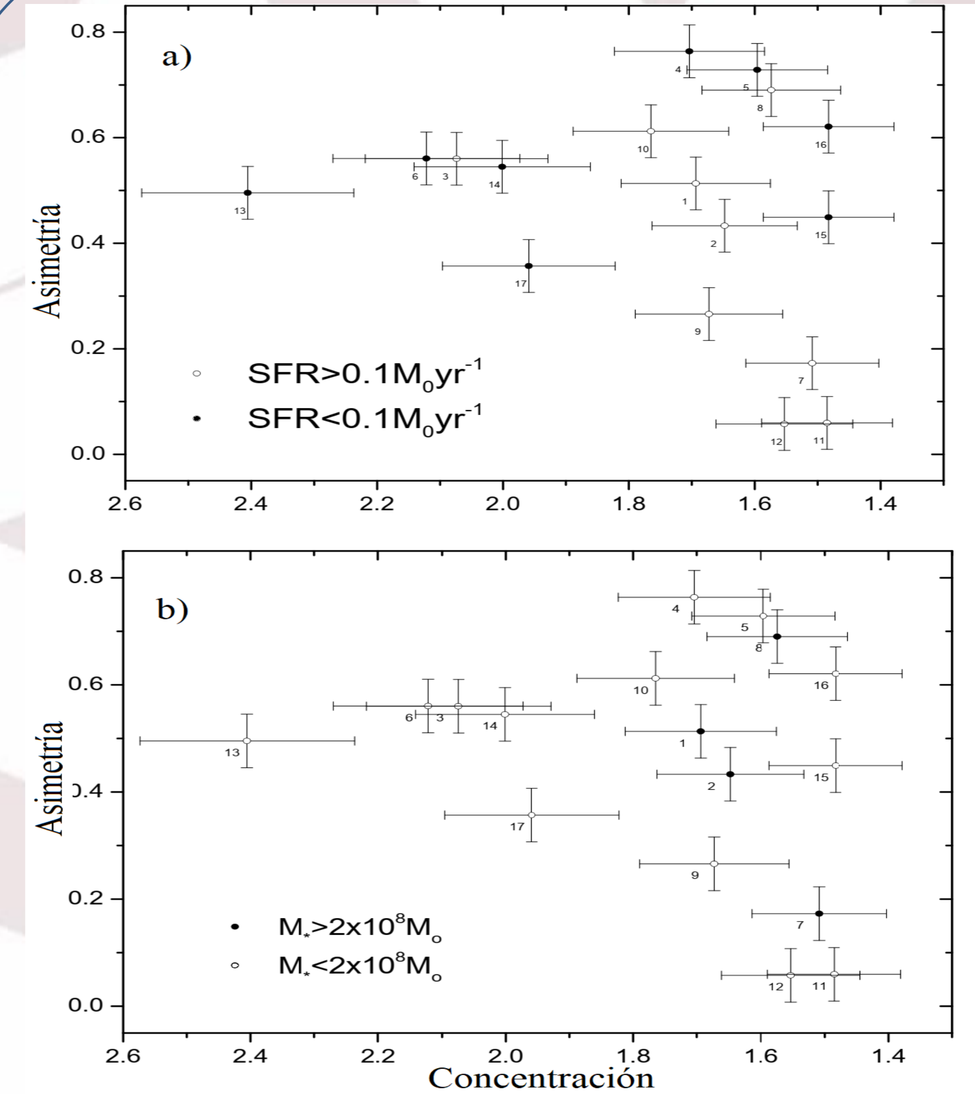
Figura 3. Plano A - C. En el panel superior a), los puntos blancos representan objetos con SFR superior a 0.1 M_{\odot} \text{yr}^{-1} , mientras que los puntos negros representan objetos con SFR inferior a 0.1 M_{\odot} \text{yr}^{-1} . En el panel inferior, los puntos negros representan objetos con una masa estelar mayor que 2 \times 10^8 M_{\odot} , y los puntos blancos representan aquellos con masa estelar menor a 2 \times 10^8 M_{\odot} .
