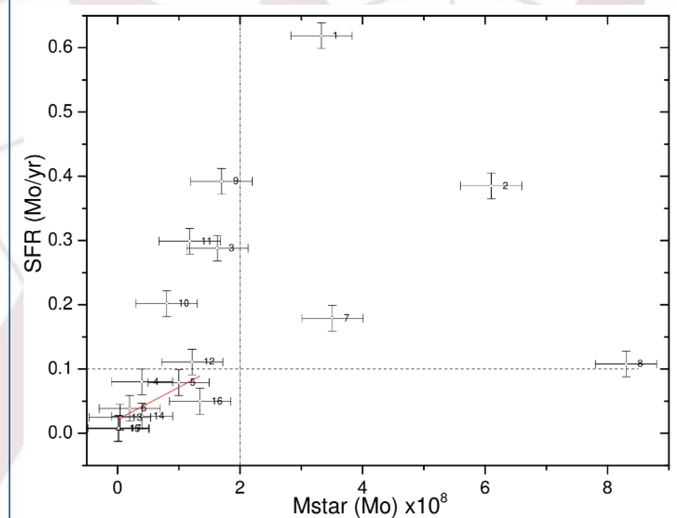
Figura 4. Tasa de formación estelar, SFR frente a la masa estelar, M_{star} . La línea discontinua horizontal representa el valor promedio de formación estelar para las galaxias enanas, y la línea discontinua vertical representa el valor promedio de la masa estelar para las galaxias enanas. La línea continua es el ajuste de los datos.
