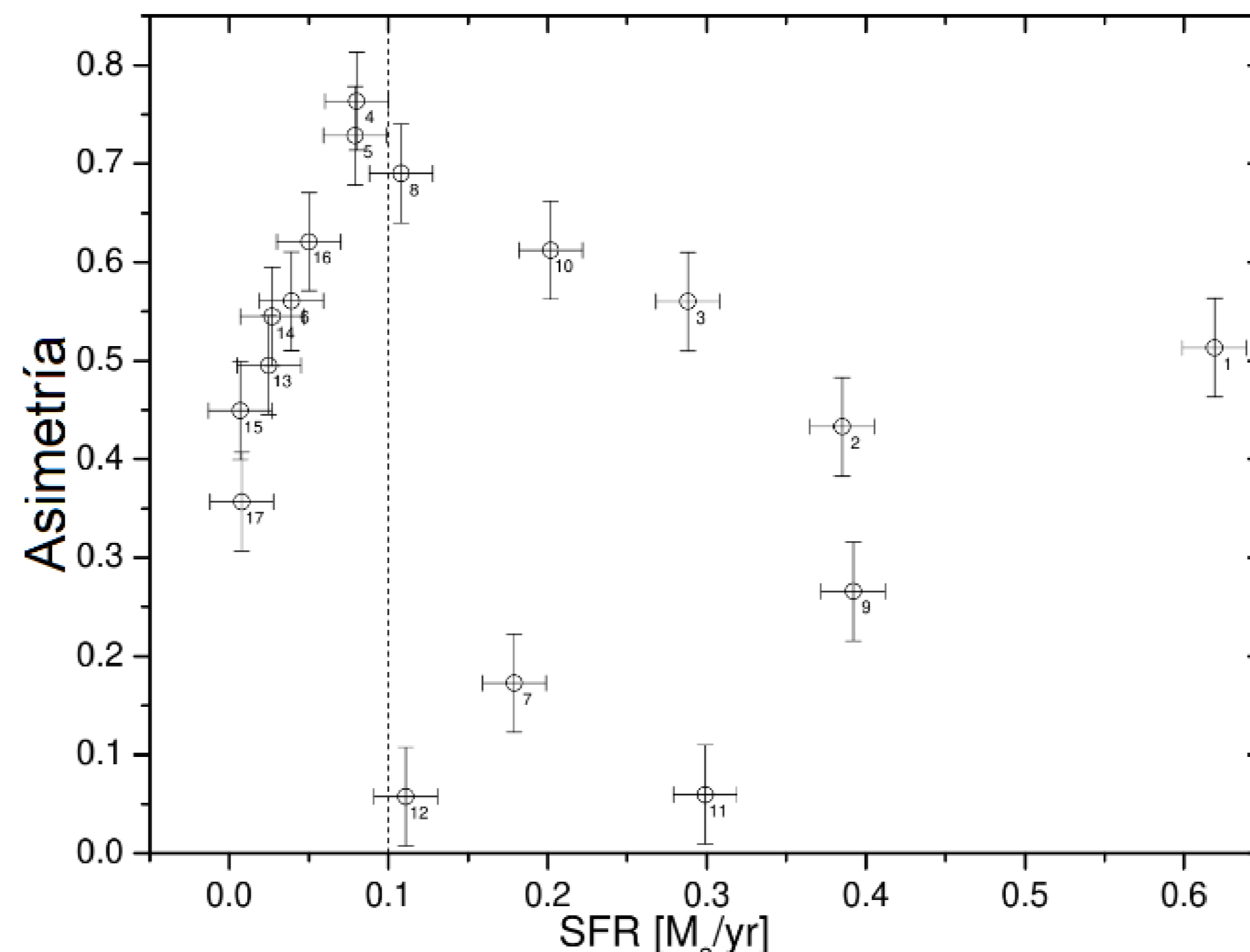
Figura 1. Asimetría frente a la tasa de formación estelar. La línea discontinua vertical representa el valor promedio de formación de estrellas para las galaxias enanas [4].
