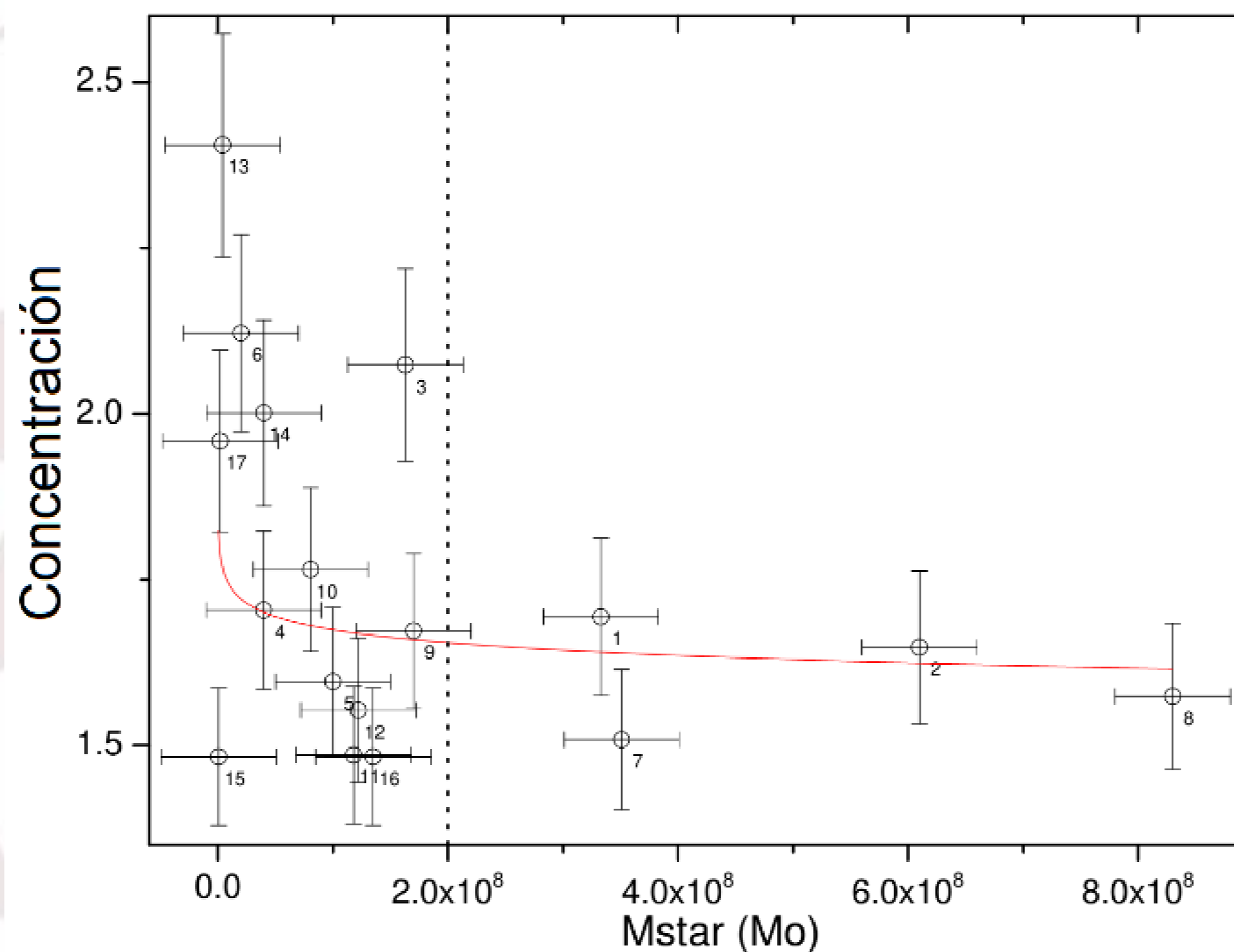
Figura 2. Concentración frente a masa estelar, M_* . La línea discontinua vertical representa el valor promedio de la masa estelar de las galaxias enanas [4], mientras que la línea continua se ajusta a los puntos de datos.
